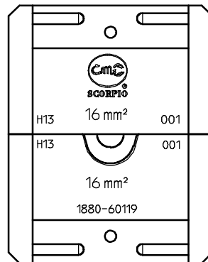
Ansicht Crimpstempel drawing view crimp punch
