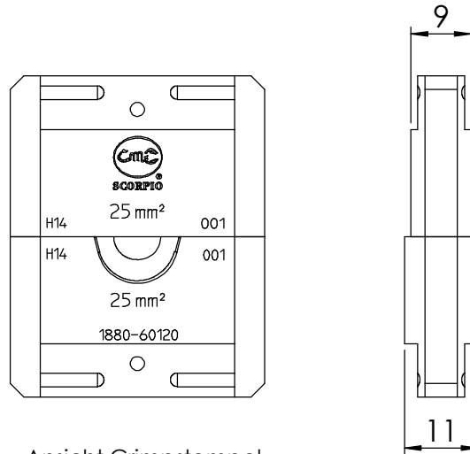
Ansicht Crimpstempel drawing view crimp punch
