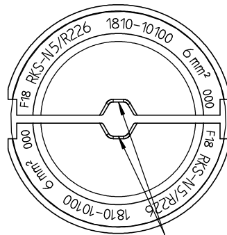
Querschnitt "6" negativ eingepreßt
